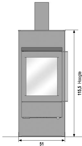
Vooraanzicht staal:
