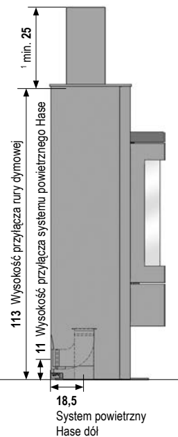
Widok z boku stal:
