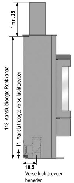
Zijaanzicht staal:
