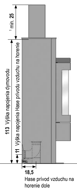
Bočný pohľad:
